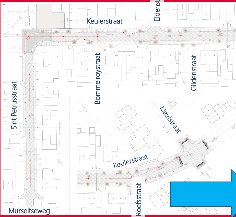
Bestaande situatie (opbreektekening)
